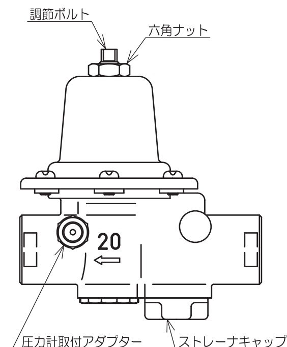
水用減圧弁 KRM・KRMA KRMAは圧力計取付アダプター付
